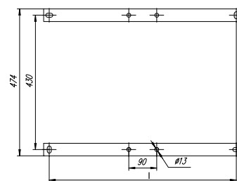
Крепление
