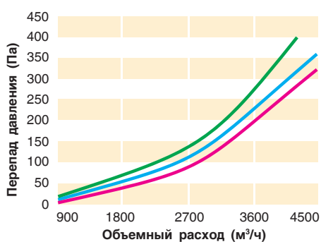
Зависимость перепада давления от объемного расхода
