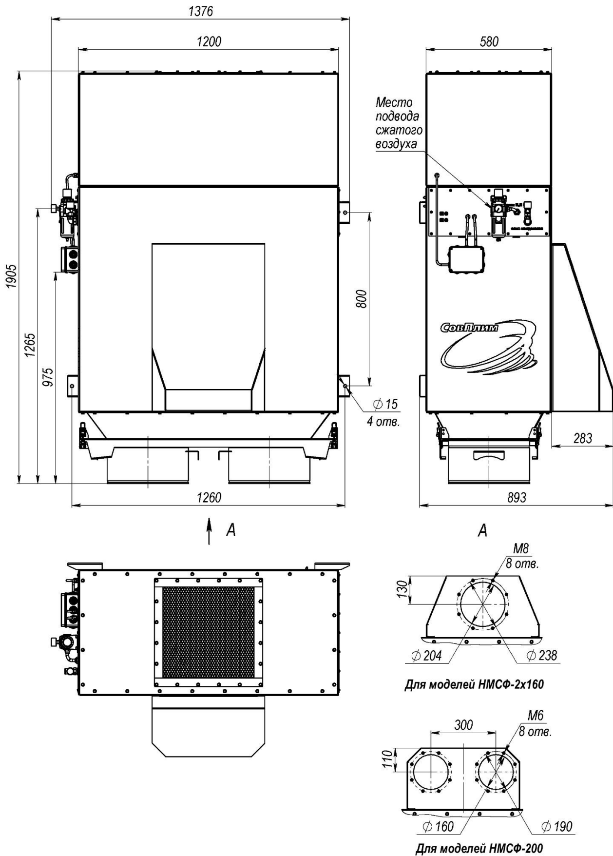
Рисунок А.1 – Габаритные и установочные размеры моделей фильтра без компрессора
