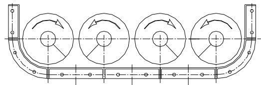
View from inlet - Ansicht von Einlauf Vue de chargement - Vista da carico
