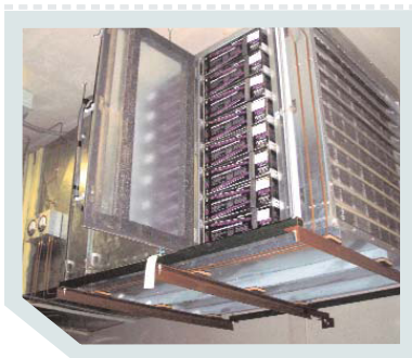
СИСТЕМА PURAFIL С БОКОВЫМ ДОСТУПОМ В УНИВЕРСИТЕТЕ В ДЖОРДЖИИ, ФАКУЛЬТЕТ ЖУРНАЛИСТИКИ
